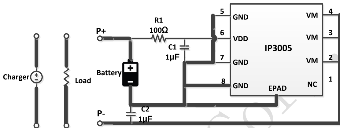
图 8 典型应用图
